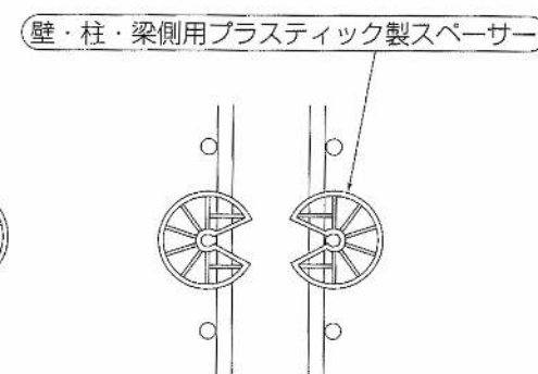
柱用プラスチック製スペーサー
