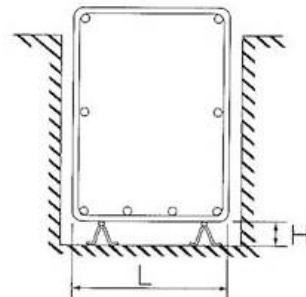
鋼製連続サポート 床スラブ下端筋用
