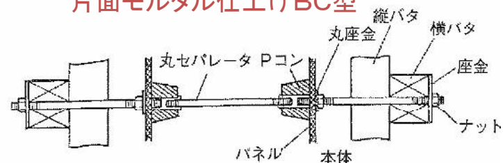
片面打ち放し 片面モルタル仕上げBC型
