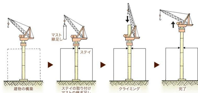
■ マストクライミング方式
