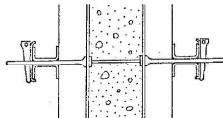
モルタル仕上げC型
