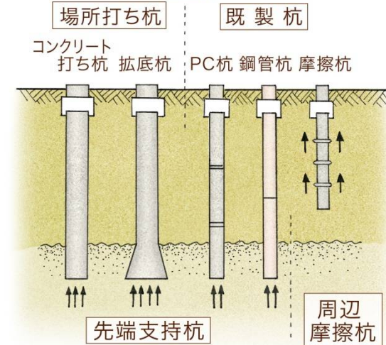
《杭の種類》
