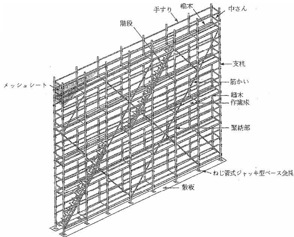
くさび緊結式足場(ビケ)
