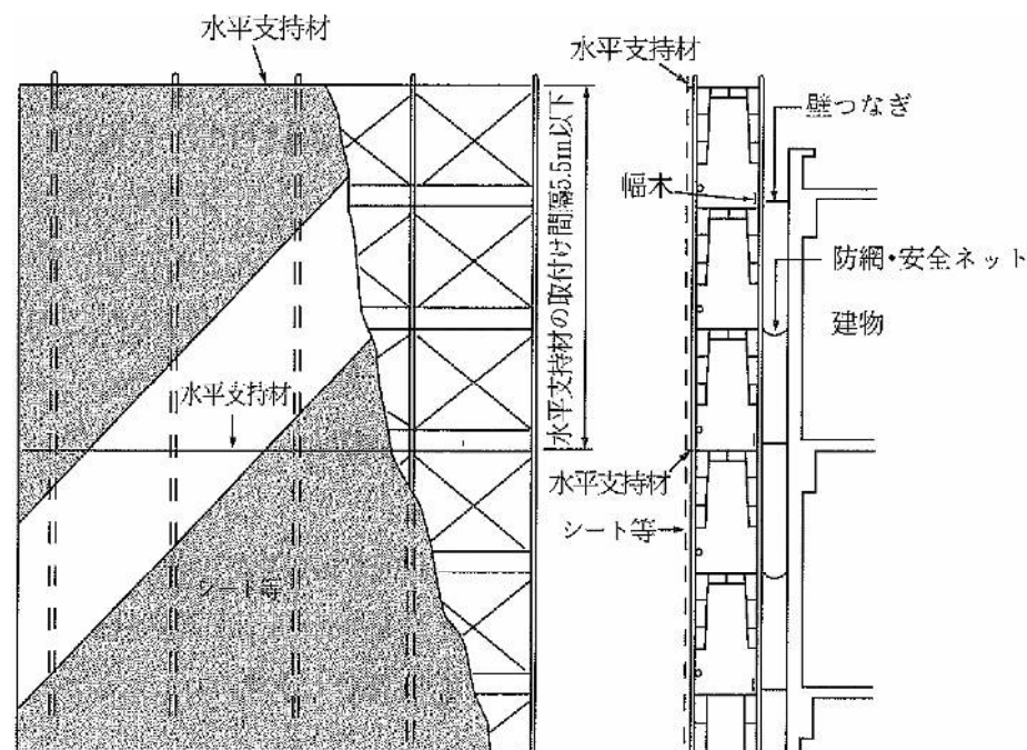
工事中シートの取付け例
