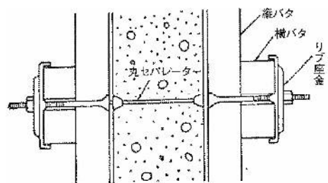
打ち放し用B型
