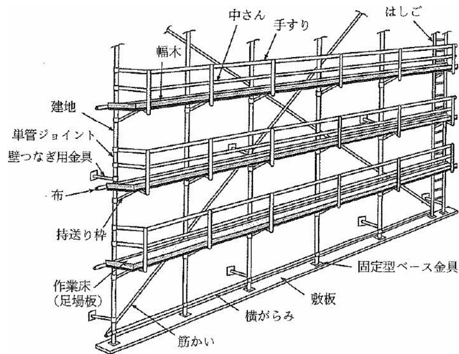
ブラケット側足場
