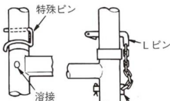
固定ピン
