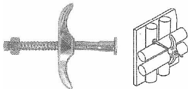
アイビーフォームタイ®3型セット
