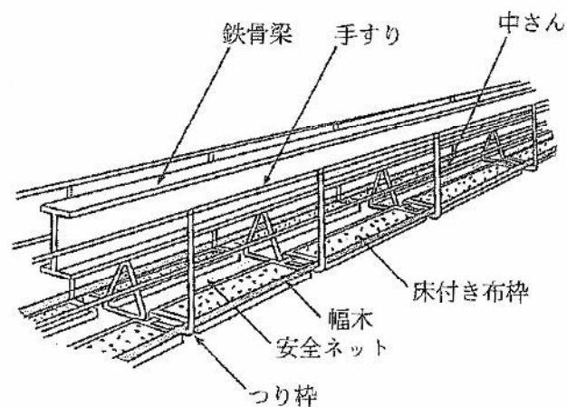
つり枠足場
