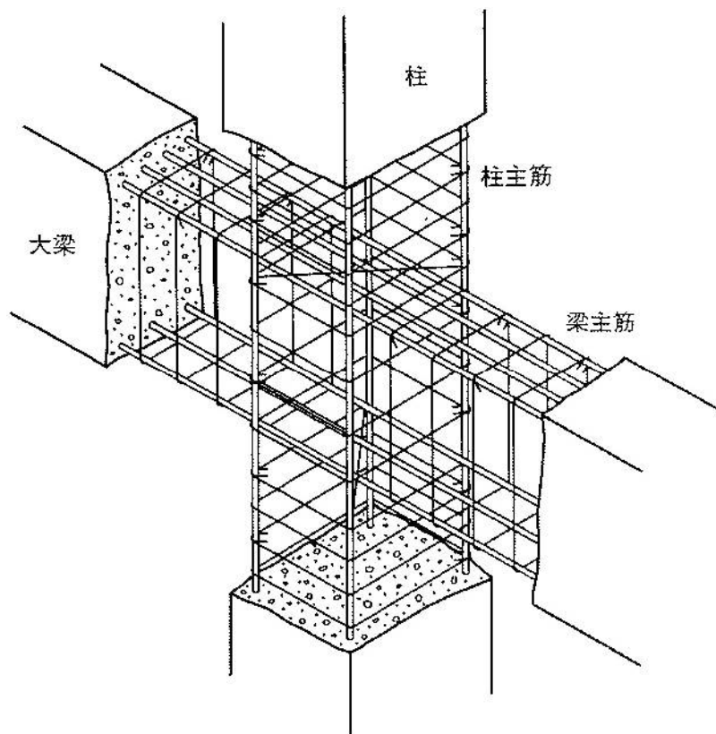
通常の内柱・梁接合部
