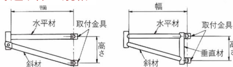
固定型開閉式
