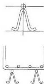
鋼製連続サポート 床スラブ下端筋用
