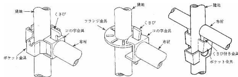
緊結方式
